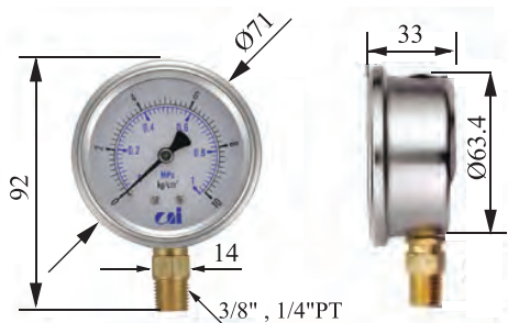
立式 LM- 60 __ kg/psi* _ / _ " PT Bottom mounting
