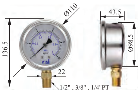
立式 LM- 100 __ kg/psi* _ / _ " PT Bottom mounting
